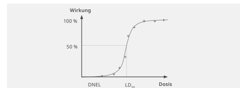
Dosis-Wirkungs-Studie „Toxizität“.
