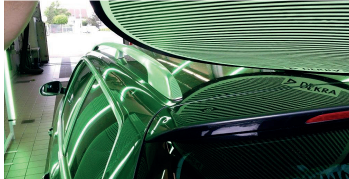
Durch den Dellenreflektor werden vorhandene Schäden sichtbar.
