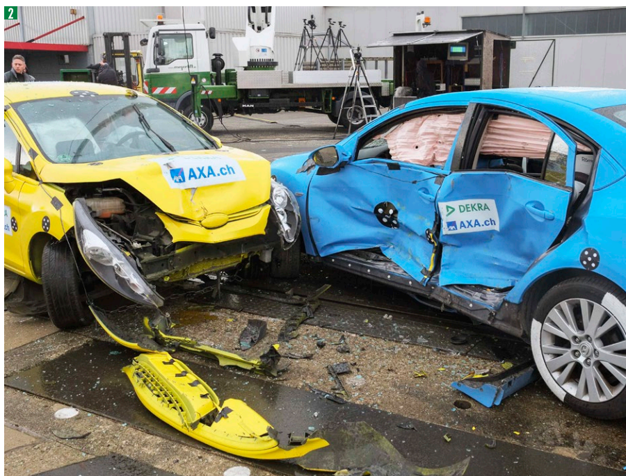
2 Ausgelöste Seitenairbags sowie stabil bleibende Schweller und B-Säule schützen den Mazda-Insassen optimal.
